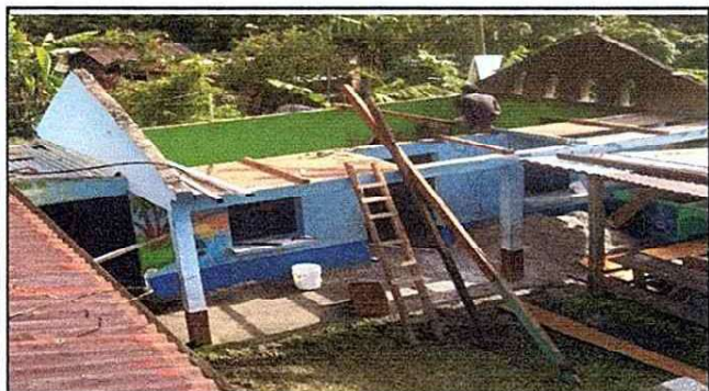
Foto 3: Desinstalación de vigas y consaneras de madera, láminas acanaladas para sustituir por estructuras metálicas y láminas troqueladas.
