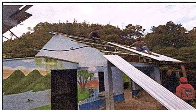
Foto 4: Instalación de estructuras metálicas y láminas troqueladas para la cocina del establecimiento educativo.
